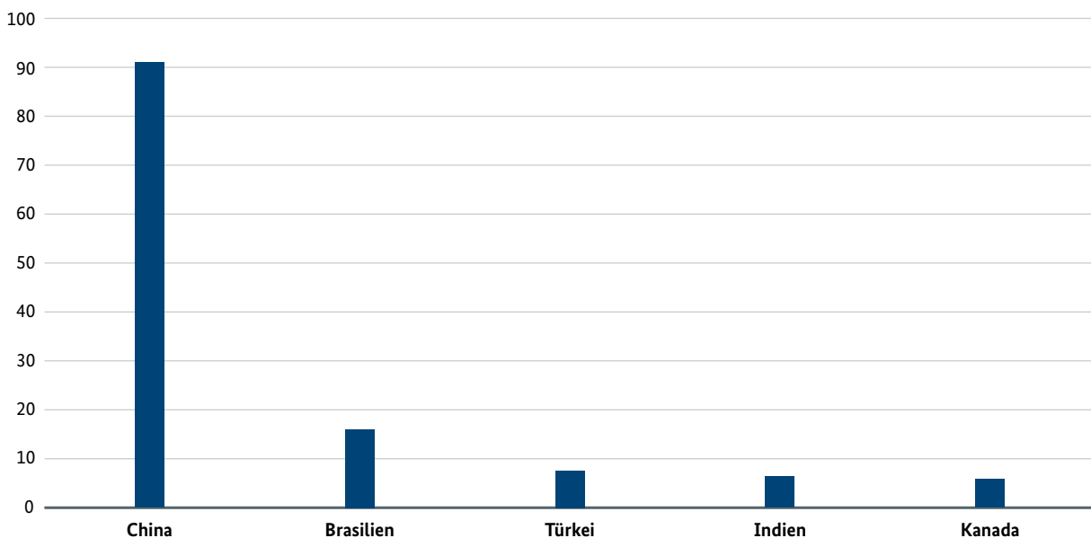
Abbildung 21: Veränderung der installierten Kapazität von Wasserkraft 2012–2017 in GW
