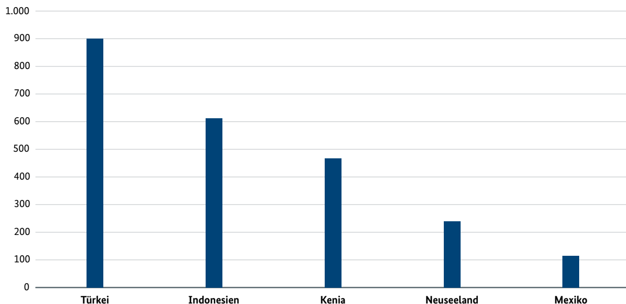
Abbildung 18: Veränderung der installierten Kapazität von Geothermieanlagen 2012–2017 in MW
