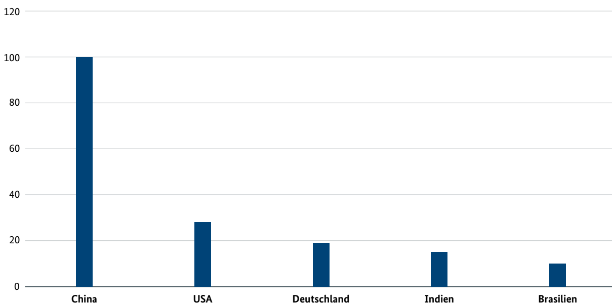
Abbildung 12: Veränderung der installierten Kapazität von Onshore Windanlagen 2012-2017 in GW
