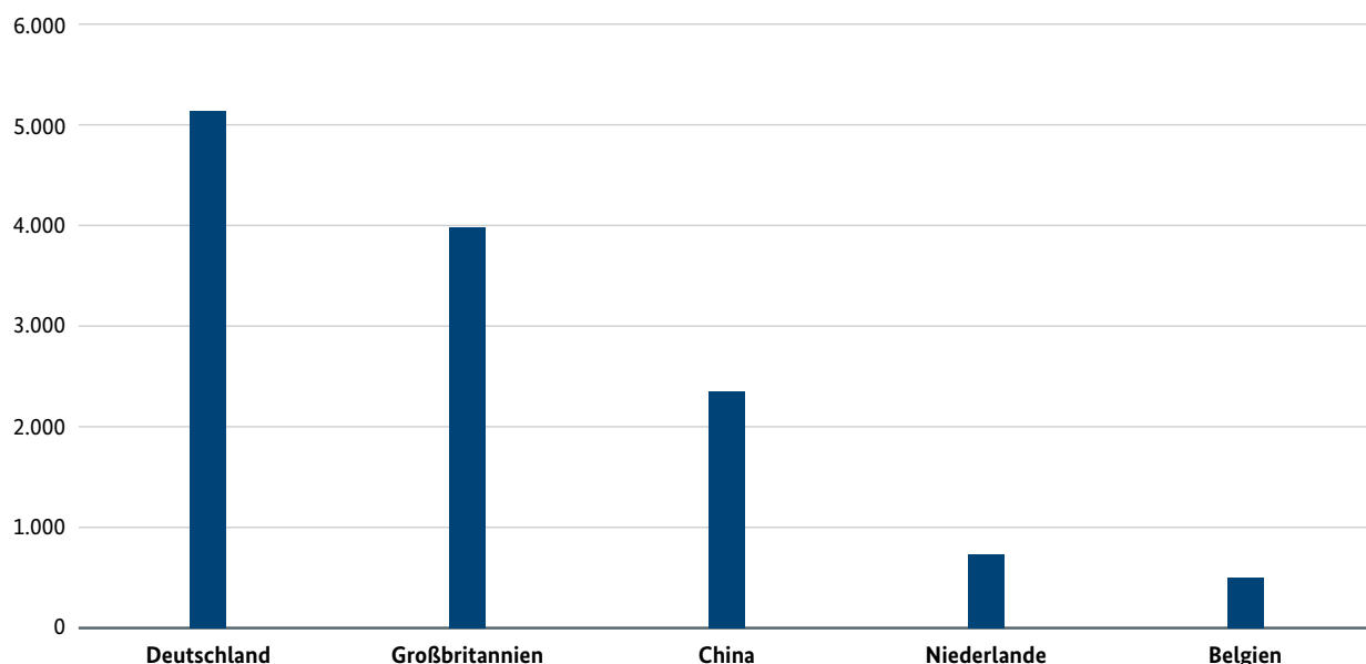
Abbildung 15: Veränderung der installierten Kapazität von Offshore Windanlagen 2012–2017 in MW
