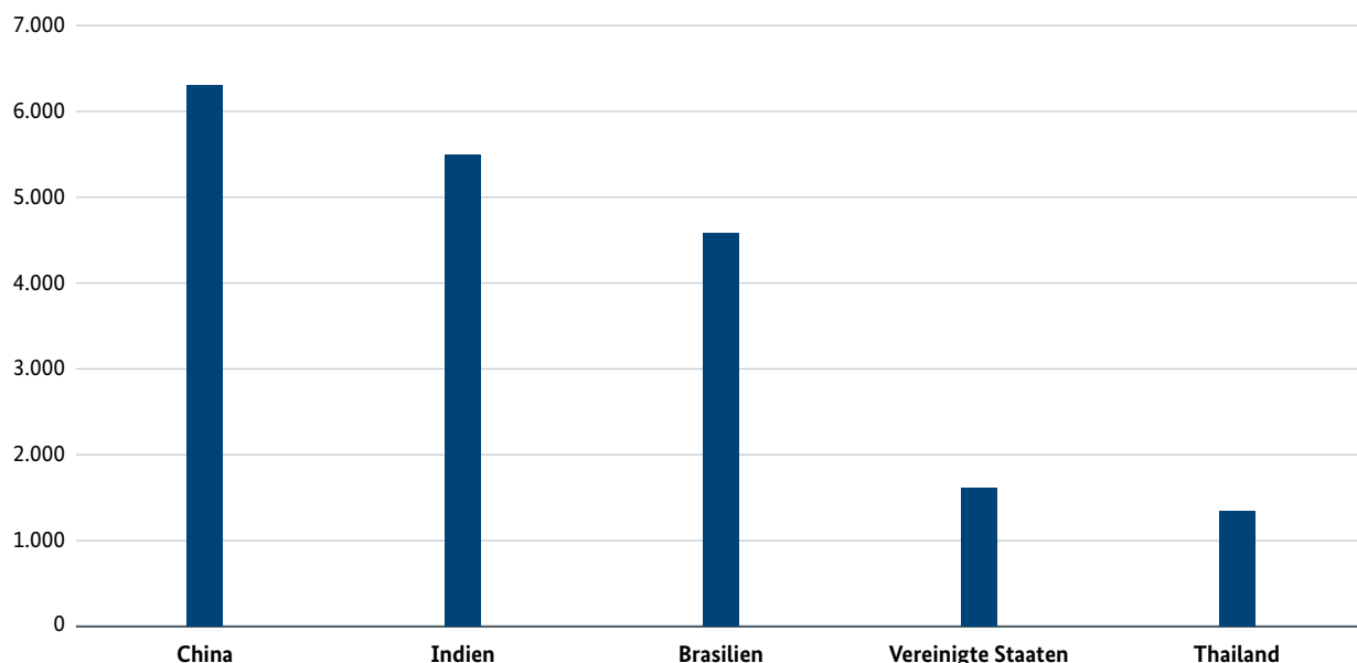
Abbildung 6: Veränderung der installierten Kapazität von feste Biomasseanlagen 2012–2017 in MW
