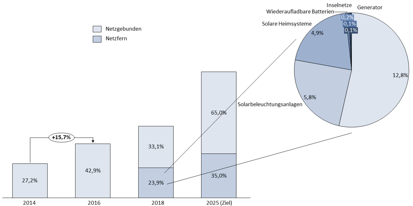
Abbildung 2: Stromversorgung, Hauptnetzzugang und netzferner Zugang
