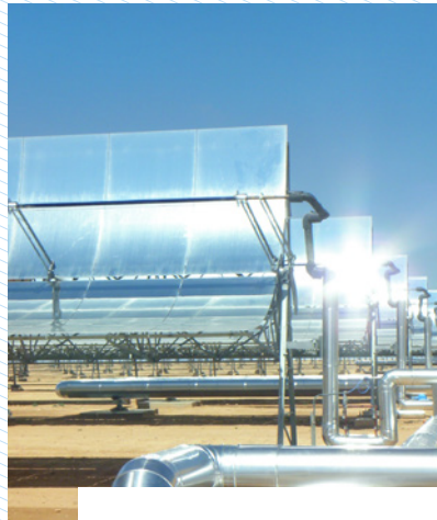
Parabolrinne (FICHTNER GMBH & CO. KG)
