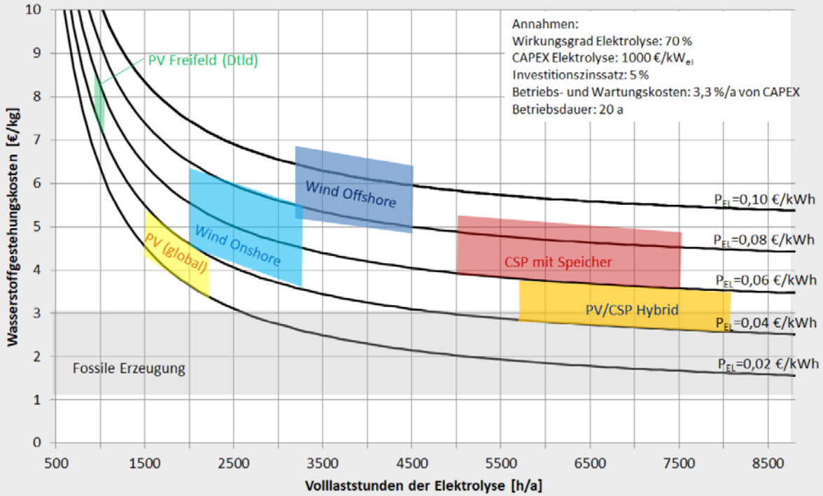
Einfluss von Volllaststunden und Stromkosten erneuerbarer Stromquellen auf die Wasserstoffgestehungskosten bei der Elektrolyse (DLR 2020)
