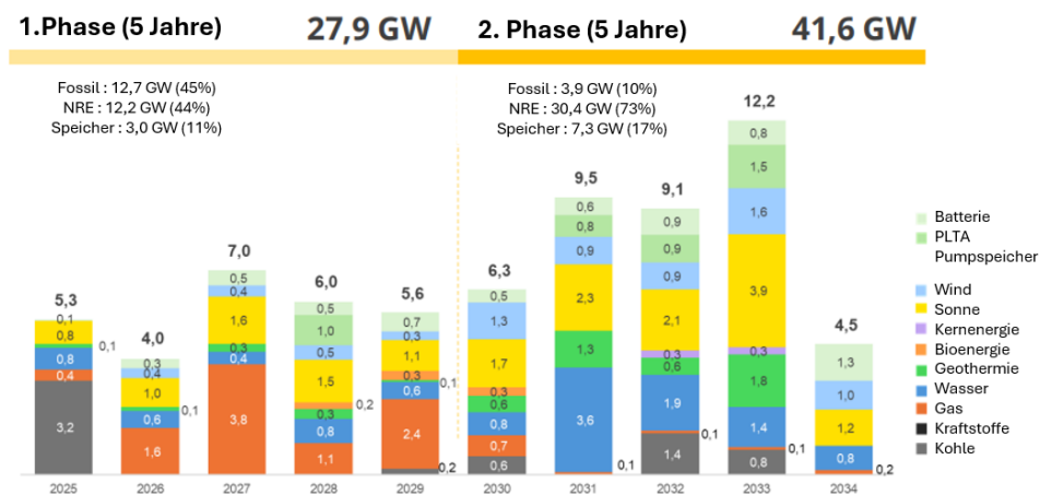
Abbildung 2: Zubau von Kraftwerkskapazitäten laut RUPTL 2025 - 2034
